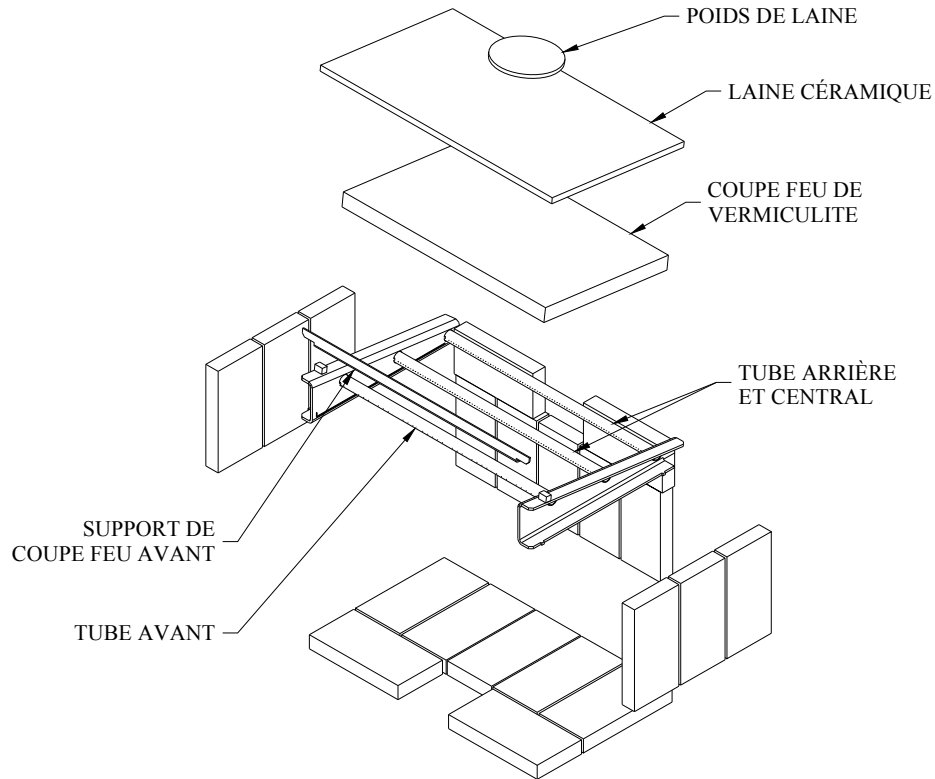
Figure 4.6.1 (A) - Installation du coupe-feu pour le modèle Escape 1800
