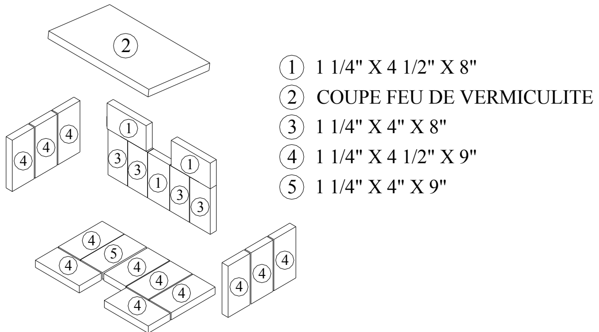
Figure 4.6.1 (B) - Disposition des briques pour le modèle Escape 1800
